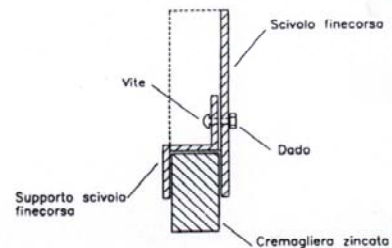
PARTICOLARE DI MONTAGGIO DEL GRUPPO FINECORSA
